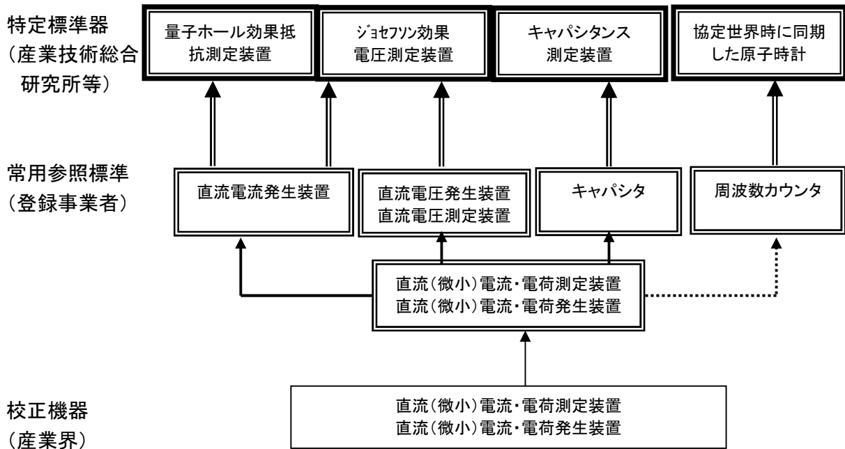
図 1-1 トレーサビリティ体系(例) <直流微小電流・電荷の場合>
