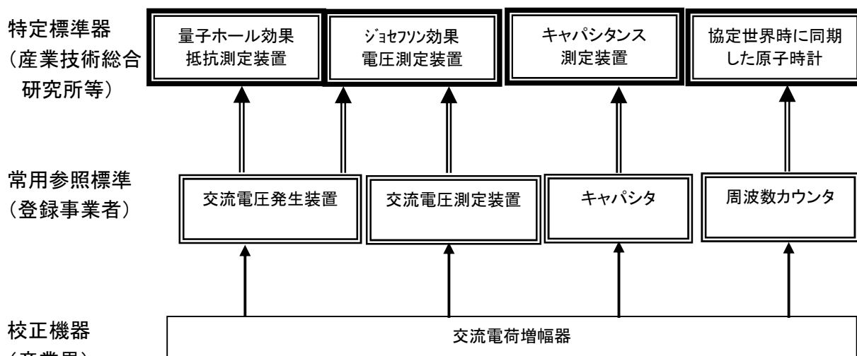
図 1-2 トレーサビリティ体系(例) &lt;交流電荷増幅器&gt;
